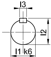
ALBERO POMPA
