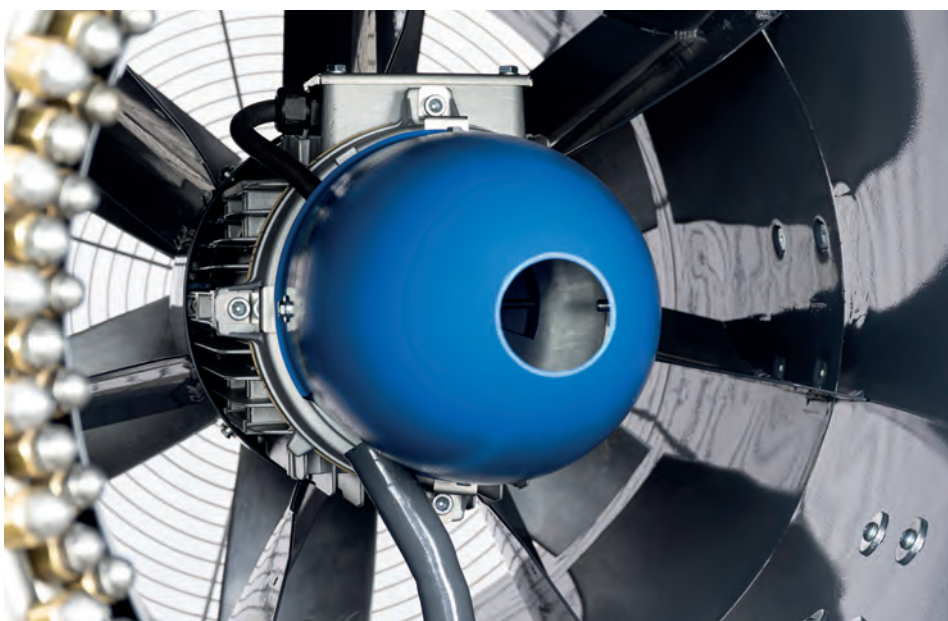
Motore ventola e configurazione dell'elica per operare a 90 metri
