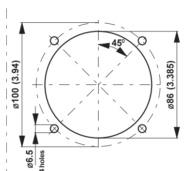
Particolari di montaggio joystick Joystick Mounting Details
